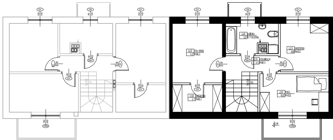
RZUT PIĘTRA
