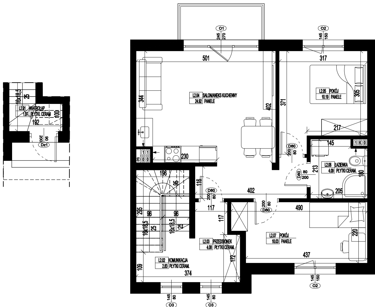
ZESTAWIENIE POW. PIĘTRA BUDYNKU E LOKALU L2
